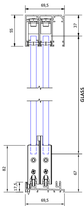
Система 2 панела
